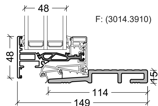
15mm threshold for 114mm frame (15mm bundstykke til 114mm karm)
