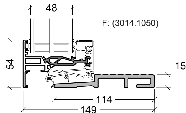
15mm threshold for 114mm frame (15mm bundstykke til 114mm karm)
