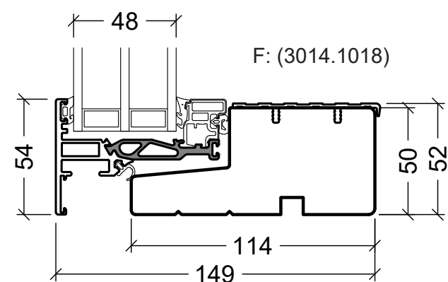
52mm threshold for 114mm frame (52mm bundstykke til 114mm karm)
