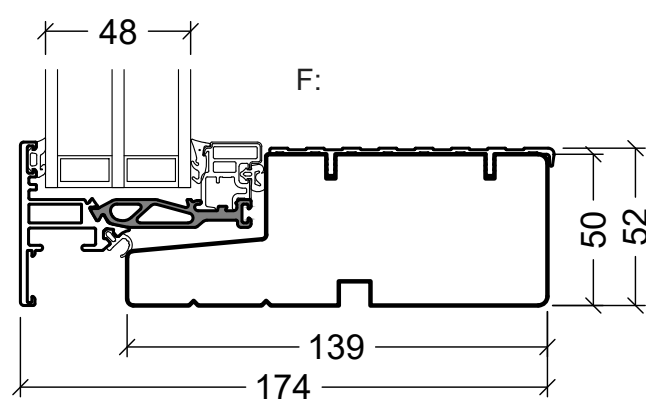
52mm threshold for 139mm frame (52 mm bundstykke til 139mm karm)
