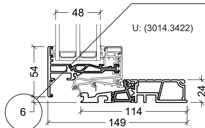
24mm threshold for 114mm frame (24mm bundstykke til 114mm karm)
