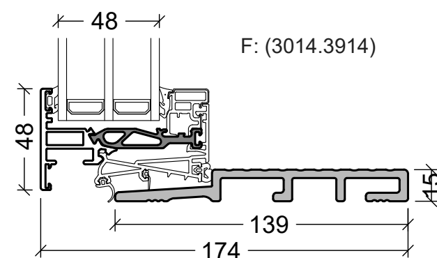
15mm threshold for 139mm frame (15mm bundstykke til 139mm karm)
