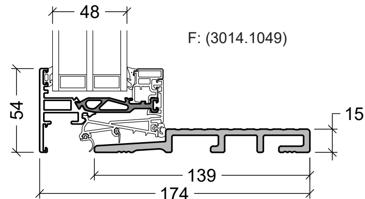
15mm threshold for 139mm frame (15mm bundstykke til 139mm karm)
