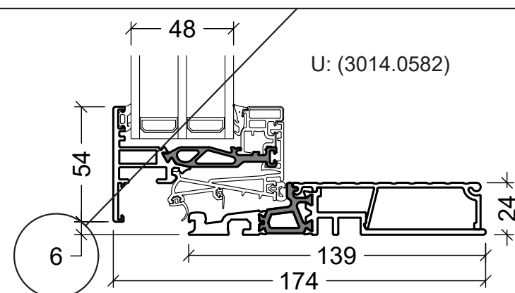
24mm threshold for 139mm frame (24mm bundstykke til 139mm karm)
